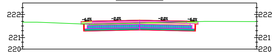
Droga 0+050.000
