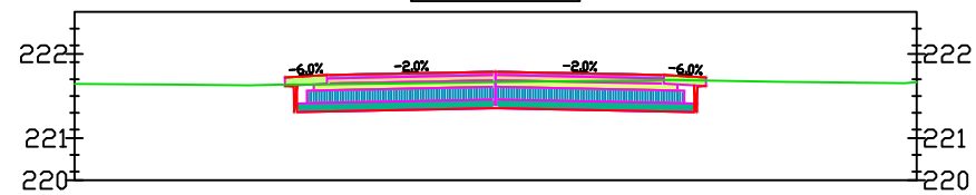
Droga 0+060.000
