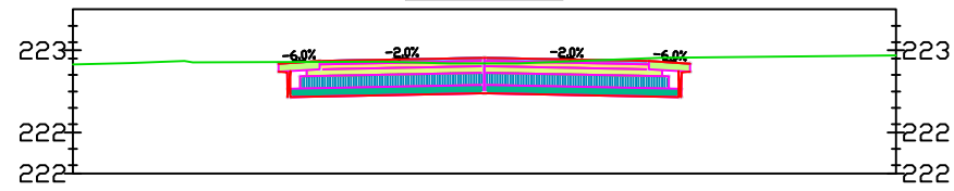
Droga 0+100.000
