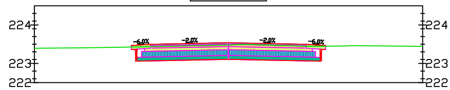
Droga 0+120.000
