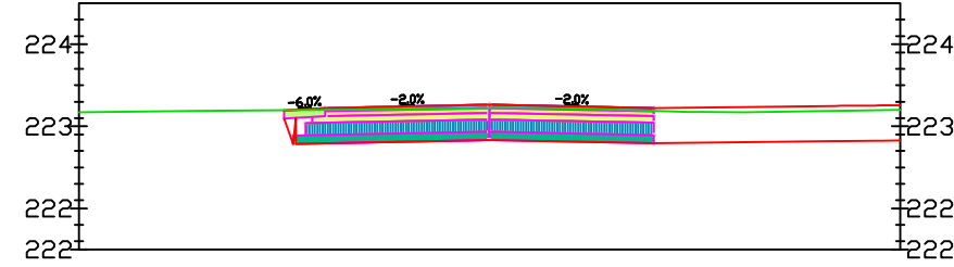
Droga 0+110.000
