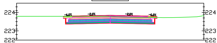
Droga 0+140.000
