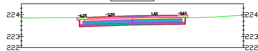
Droga 0+150.000
